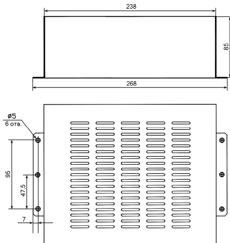
Рисунок 2 - Габаритные размеры защитного кожуха
